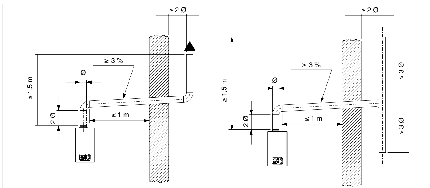
Εικ. 6 Συνδέσεις στην καπνοδόχο των μοντέλων με ανοιχτό θάλαμο
