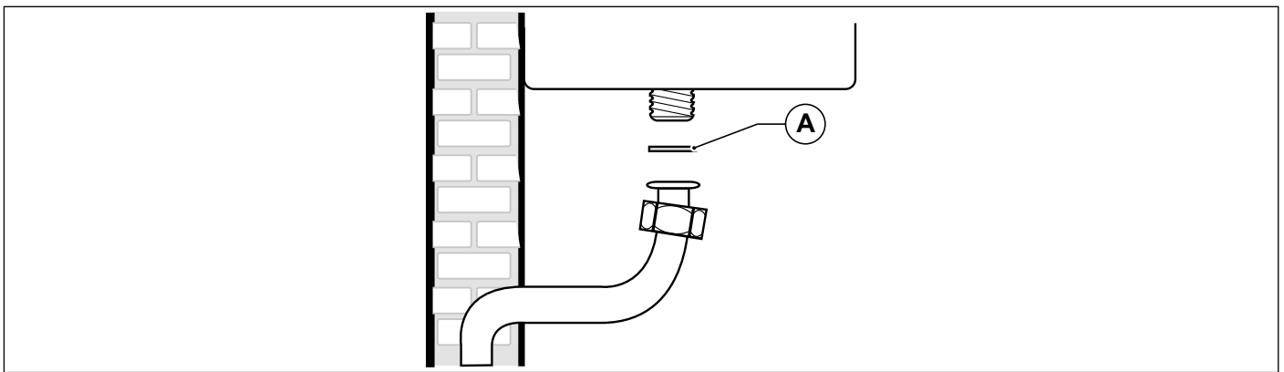
Εικ. 8 Σύνδεση με το δίκτυο αερίου
