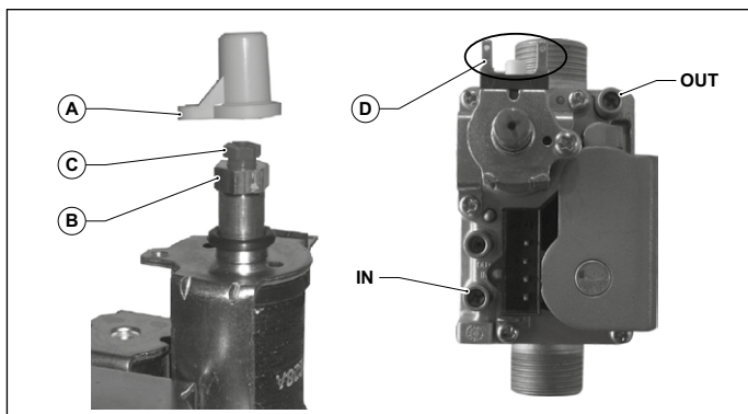
Εικ. 13 SIEMENS VGUS56
