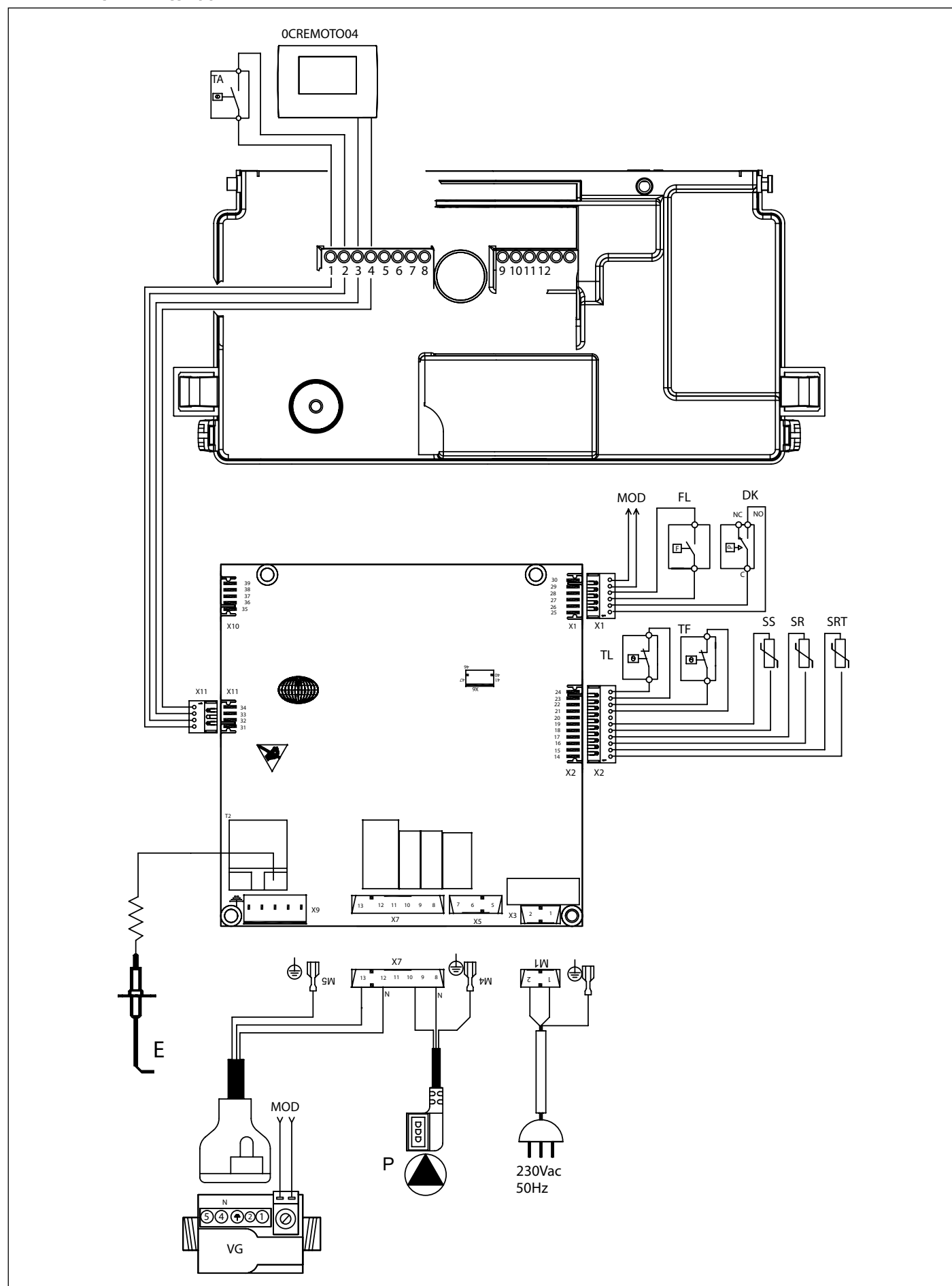
Εικ. 10 Ηλεκτρικό διάγραμμα
