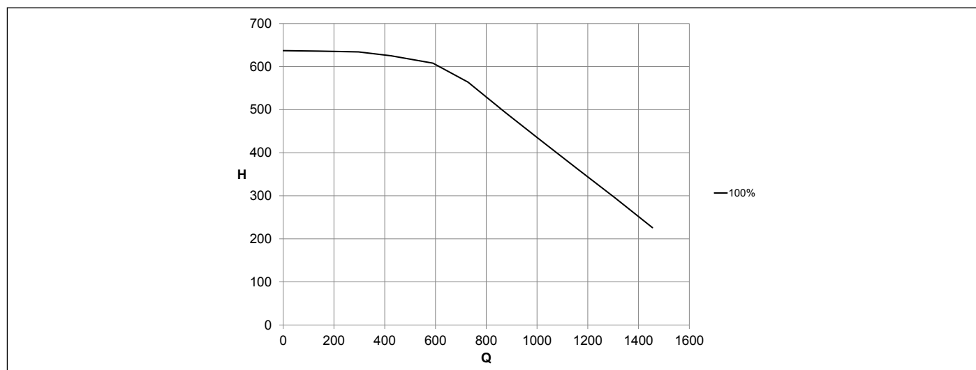
Εικ. 9 Διαθέσιμη αντίσταση
