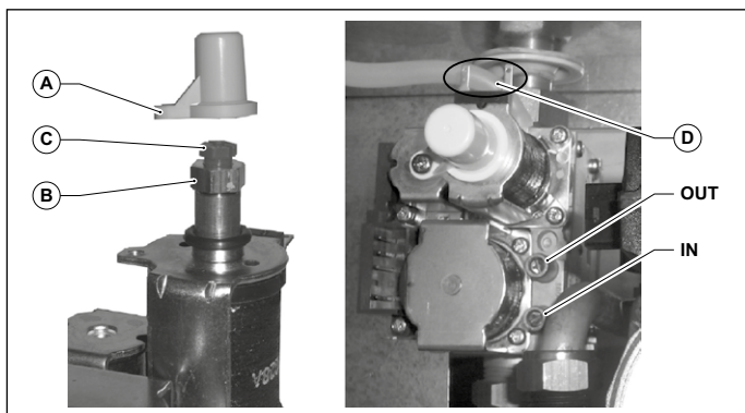
Εικ. 11 SIEMENS VGU56
