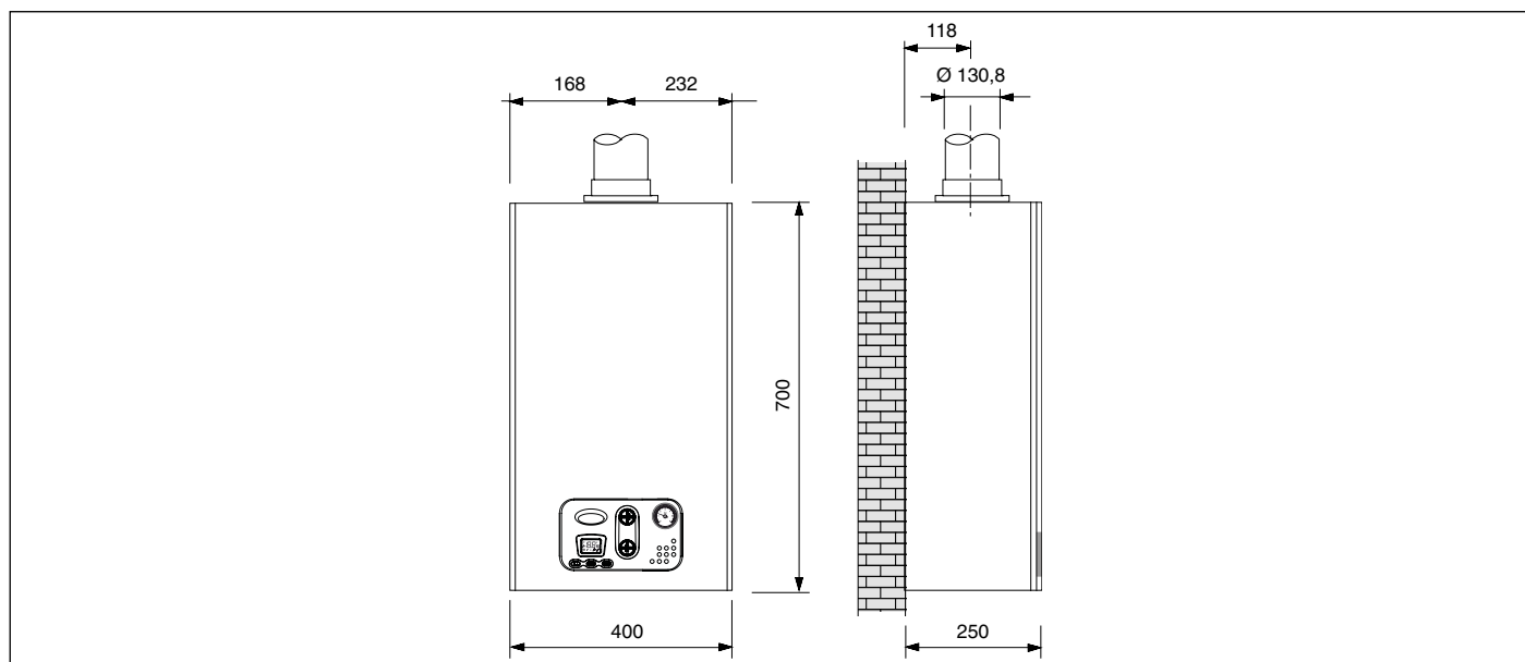
Εικ. 7 Διαστασιολογήσεις για τη σύνδεση αγωγού εκκένωσης καπνού των μοντέλων με ανοιχτό θάλαμο
