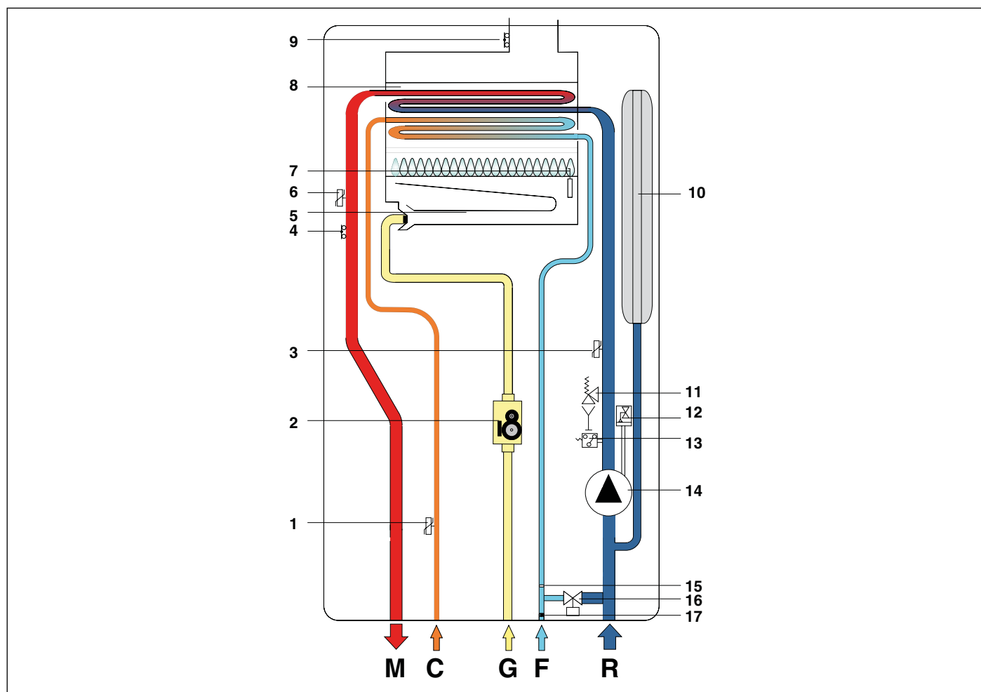
Εικ. 4 Υδραυλικό διάγραμμα CTN
