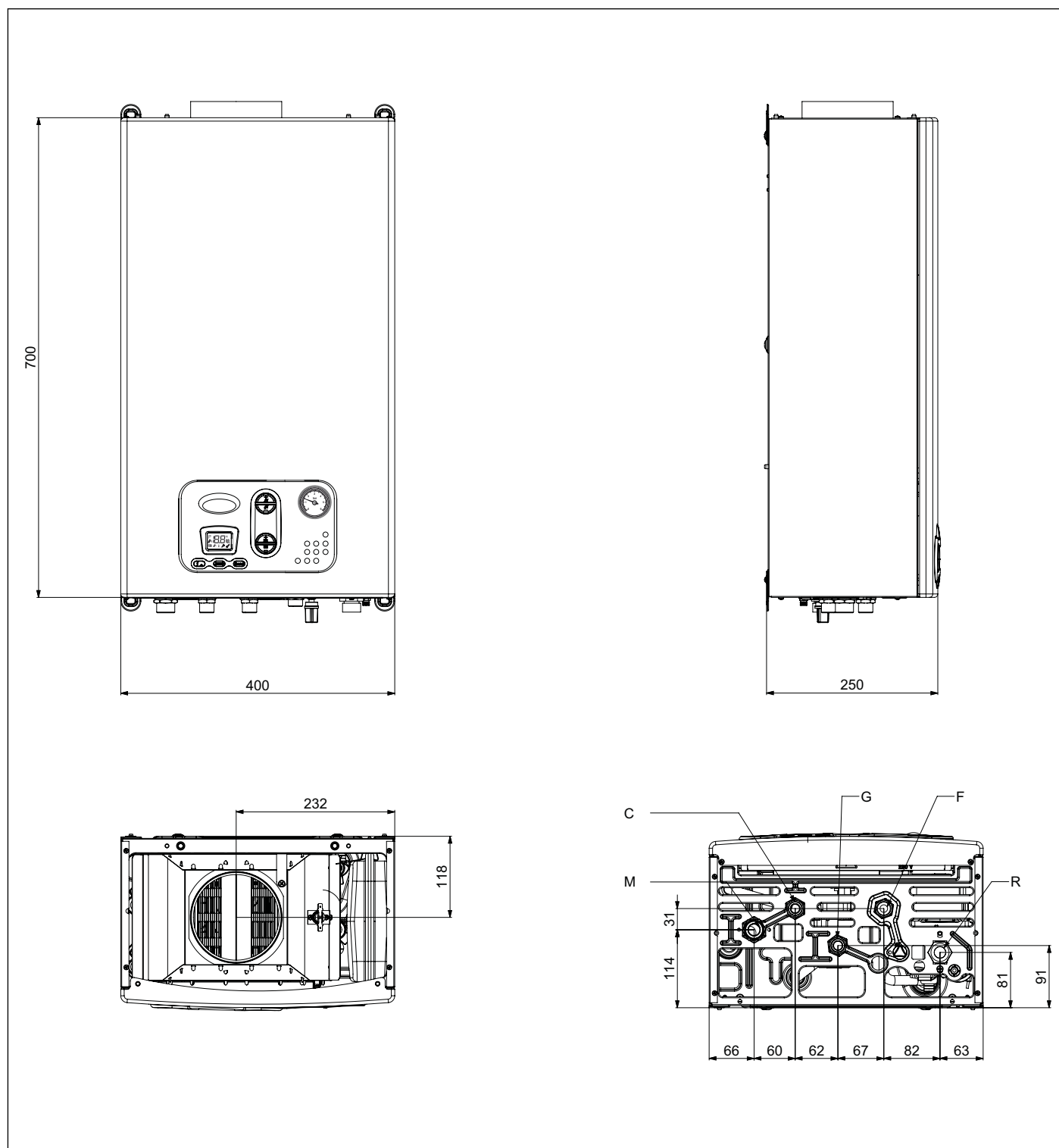
Εικ. 3 Διαστάσεις CTN
