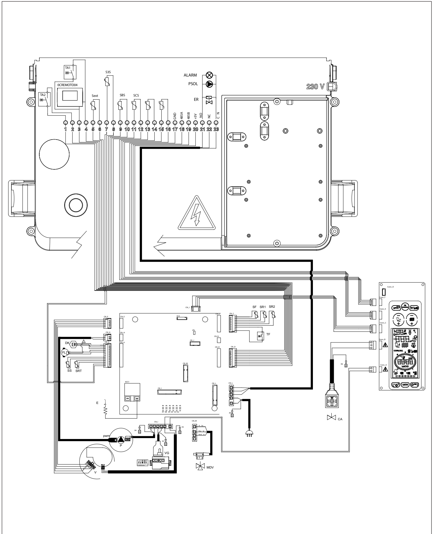
Εικ. 24 Ηλεκτρικό διάγραμμα KC
