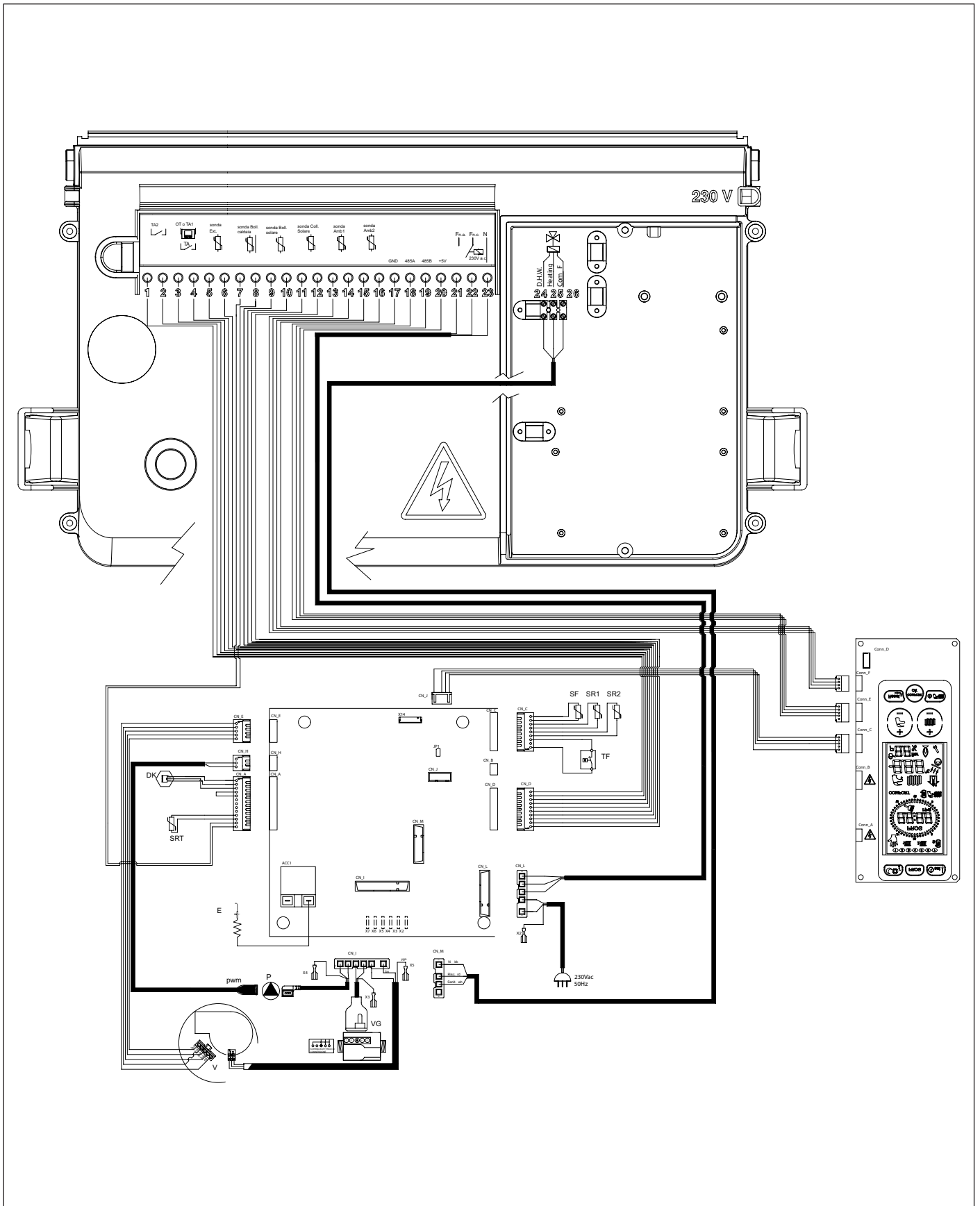
Εικ. 29 Ηλεκτρικό διάγραμμα KR
