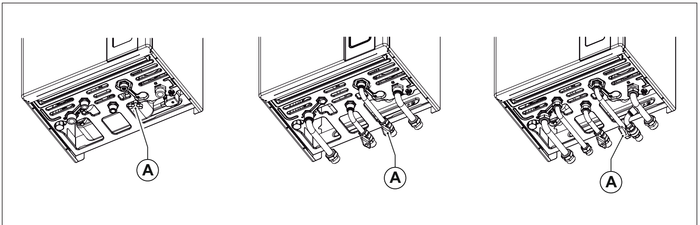
Εικ. 2 Βάνες φόρτωσης
