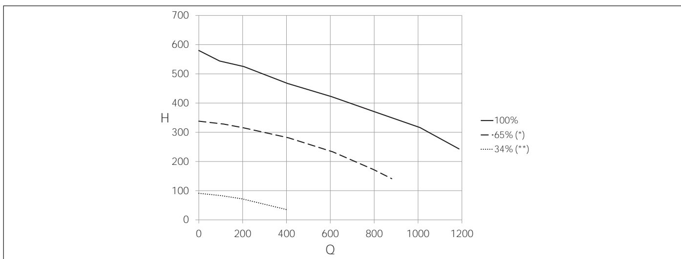
Εικ. 22 Διαθέσιμη αντίσταση KC-KR-KRB 28
