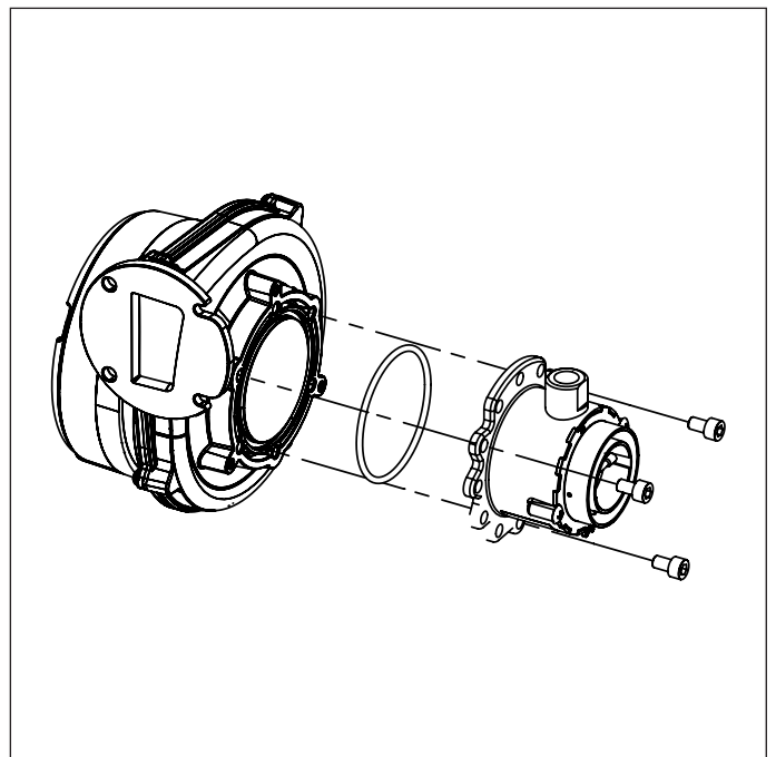
Εικ. 37 Μείκτης
