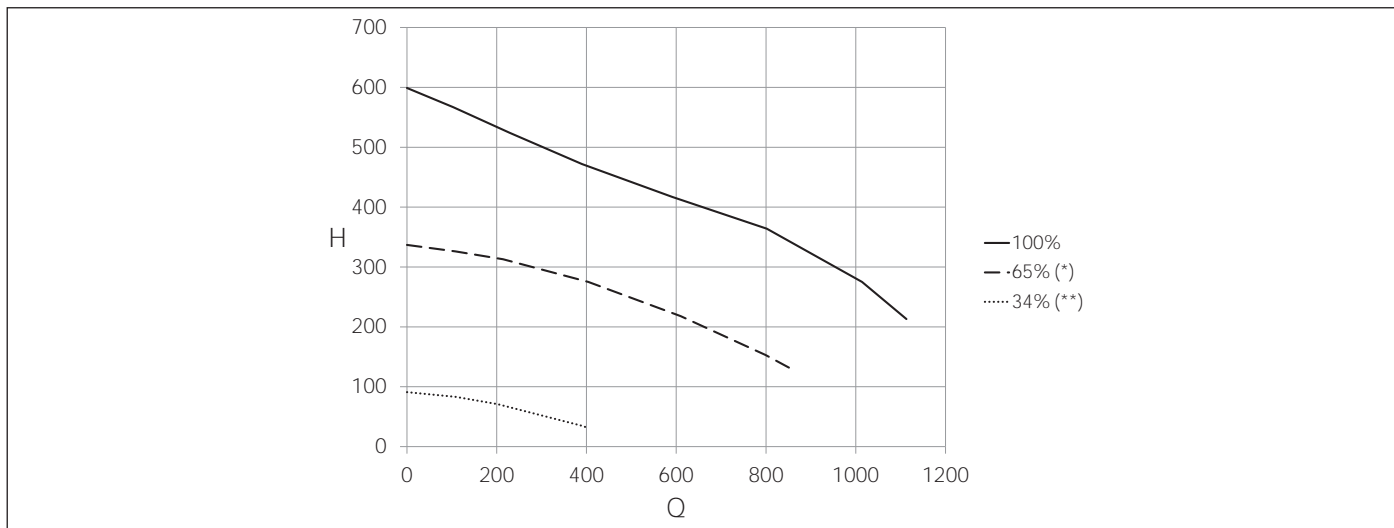
Εικ. 21 Διαθέσιμη αντίσταση KC-KR-KRB 24
