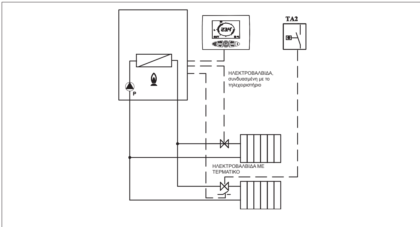
Εικ. 33 Ρελέ με τηλεχειριστήριο και TA2
