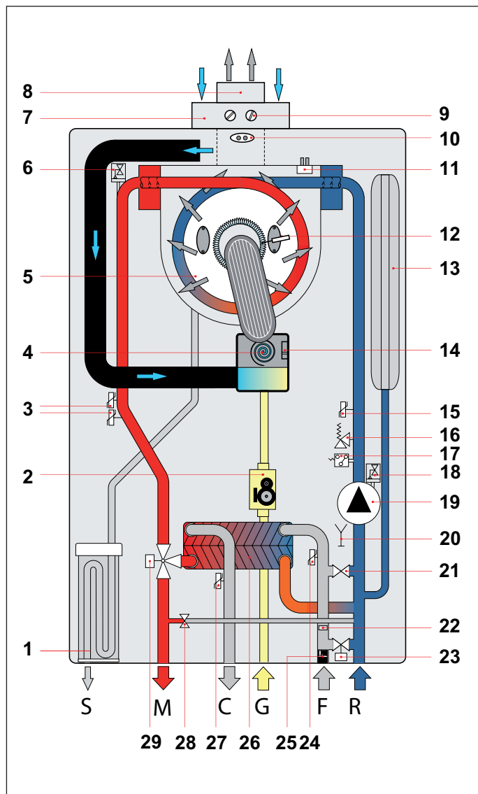
Εικ. 6 Υδραυλικό διάγραμμα μοντέλου ΚC
