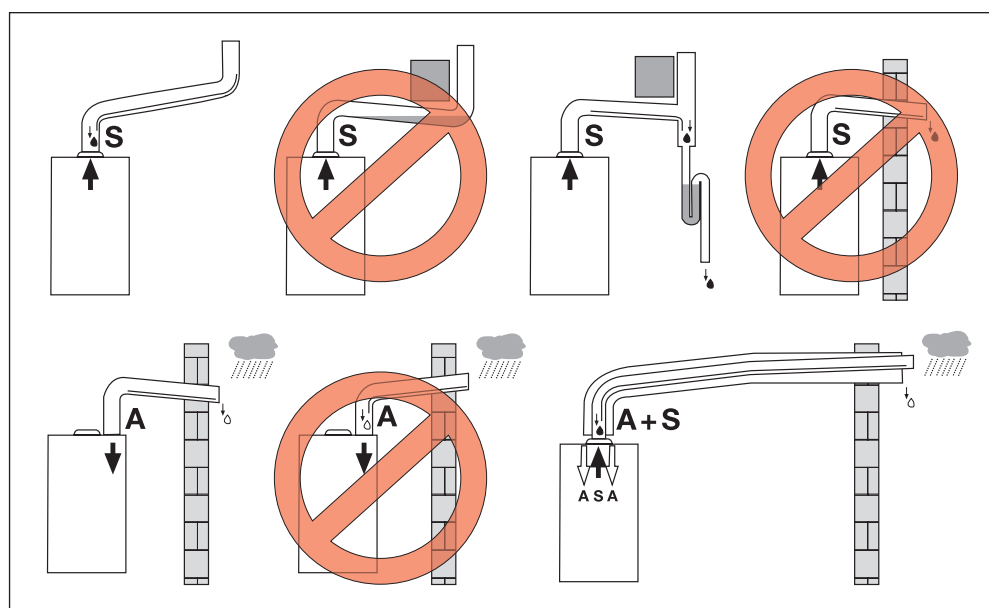
Εικ. 10 Παραδείγματα εγκατάστασης
