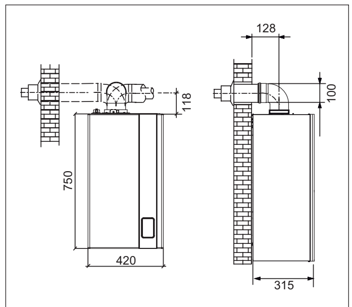
Εικ. 12 Διαστάσεις ομοαξονικών αγωγών τύπου C33
