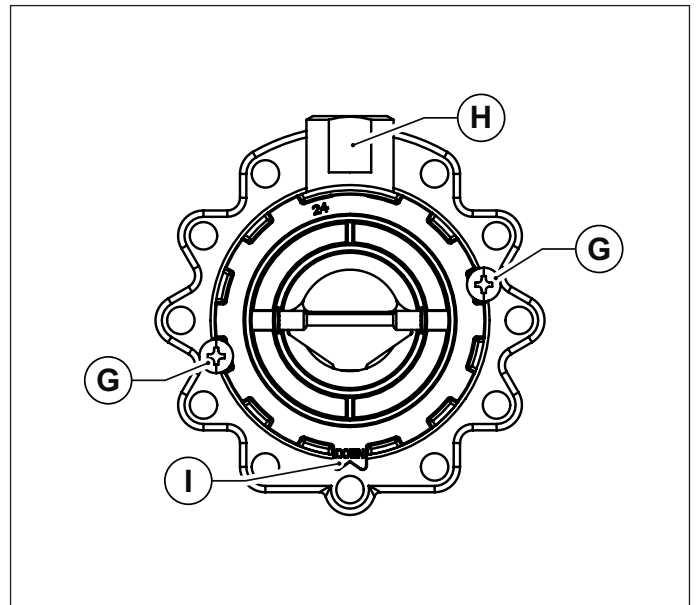
Εικ. 39 Προσανατολισμός συναρμολόγησης
