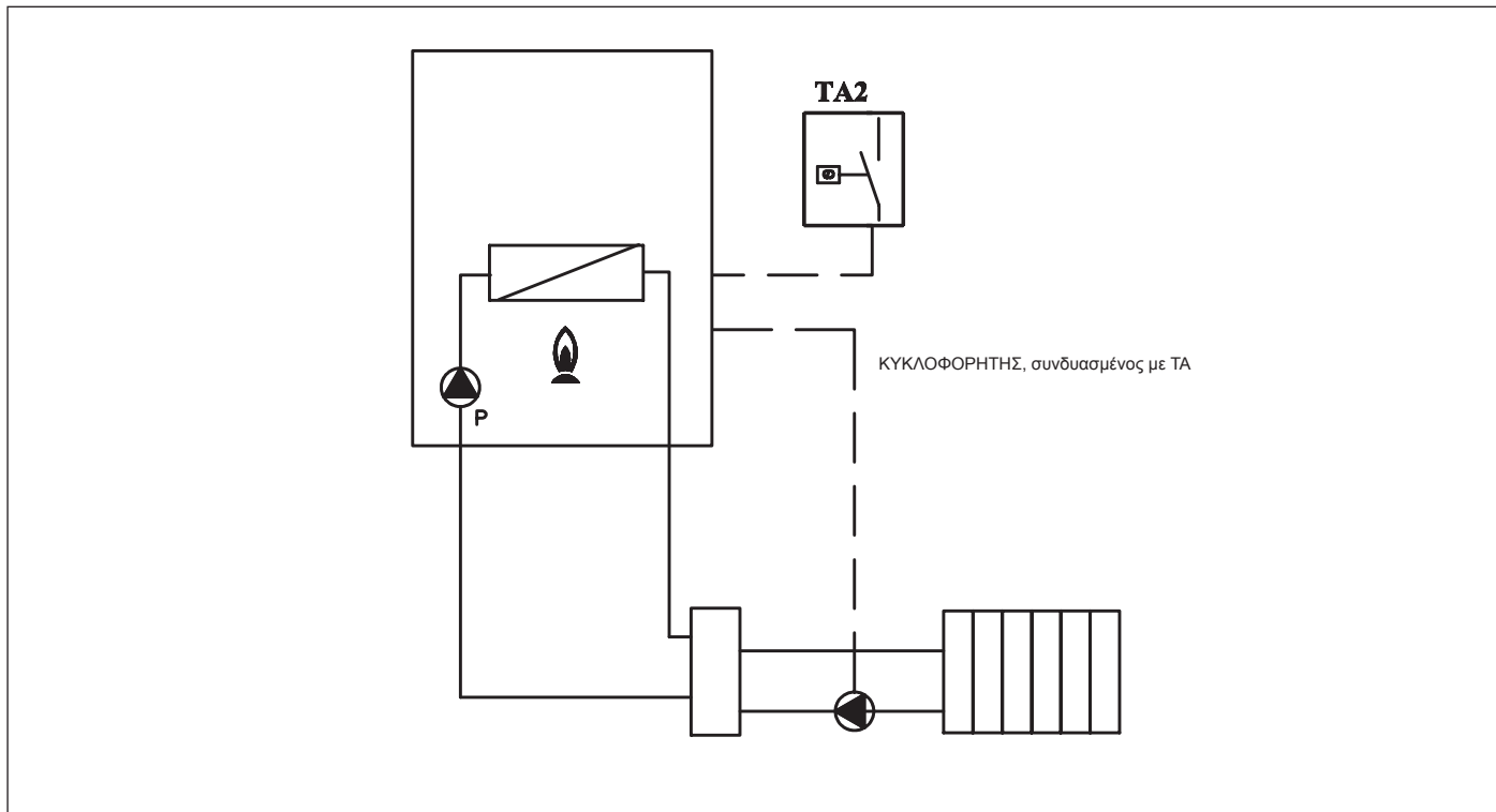
Εικ. 35 Ρελέ με αίτημα (P17=3)
