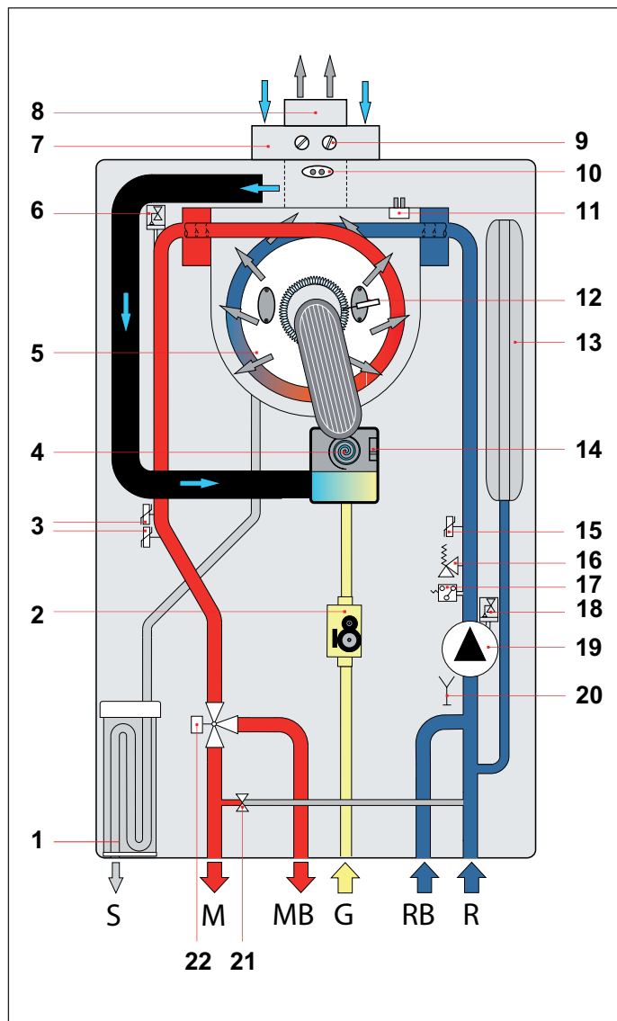
Εικ. 8 Υδραυλικό διάγραμμα μοντέλου KRB
