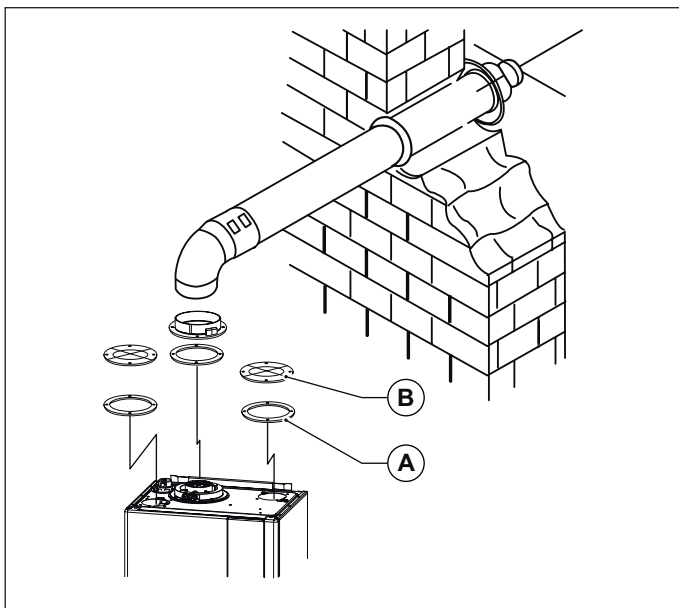
Εικ. 11 Ομοαξονικοί αγωγοί τύπου C33
