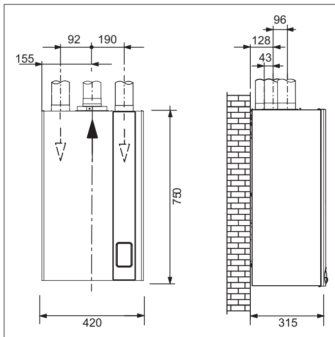
Εικ. 14 Διαστάσεις ομοαξονικών αγωγών τύπου C43 - C53 - C83
