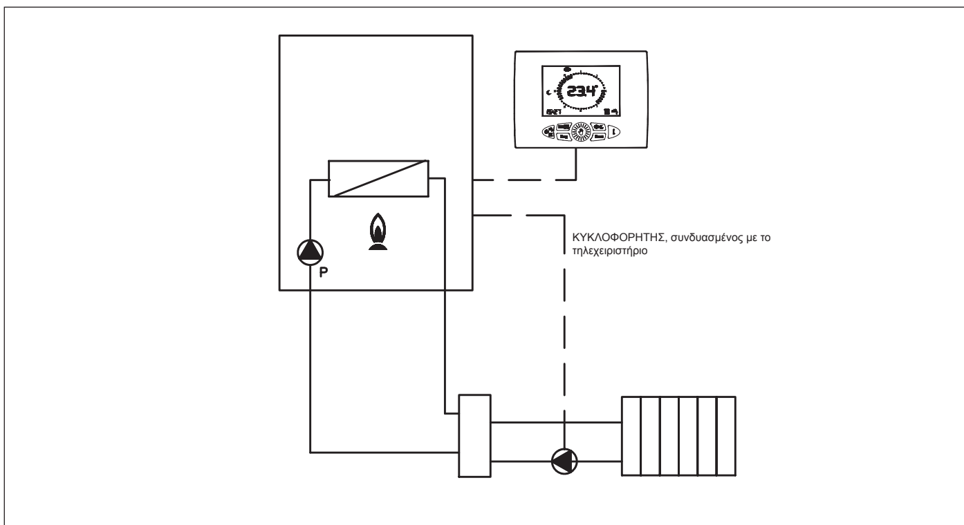
Εικ. 34 Ρελέ με αίτηση τηλεχειριστηρίου (P17=1)
