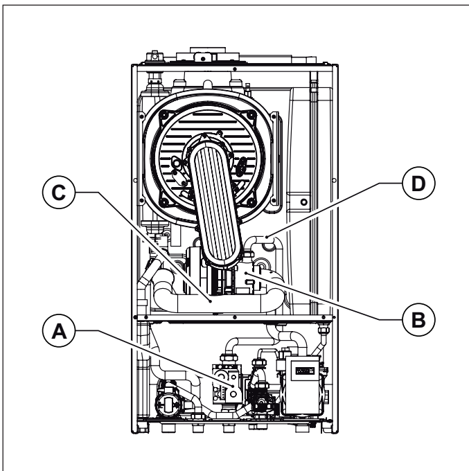
Εικ. 36 Εξάτμιση αναρρόφησης
