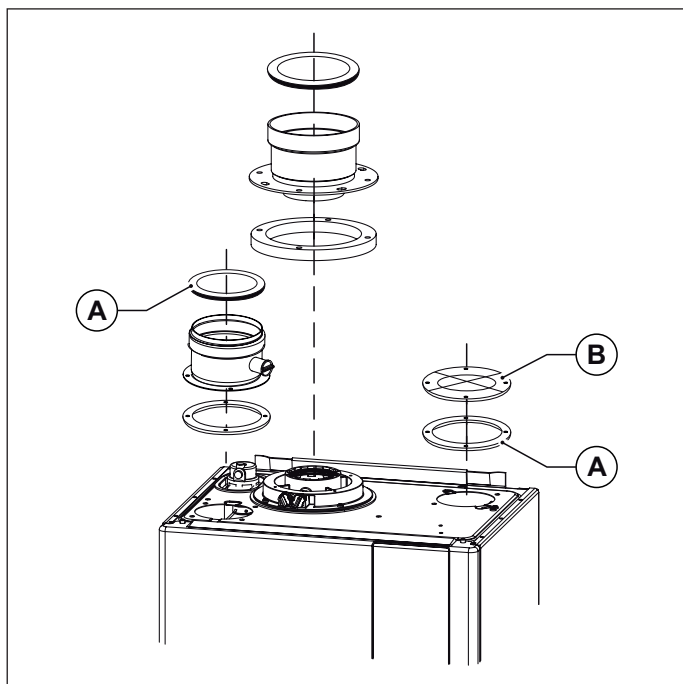
Εικ. 13 Διαστάσεις ομοαξονικών αγωγών τύπου C43 - C53 - C83
