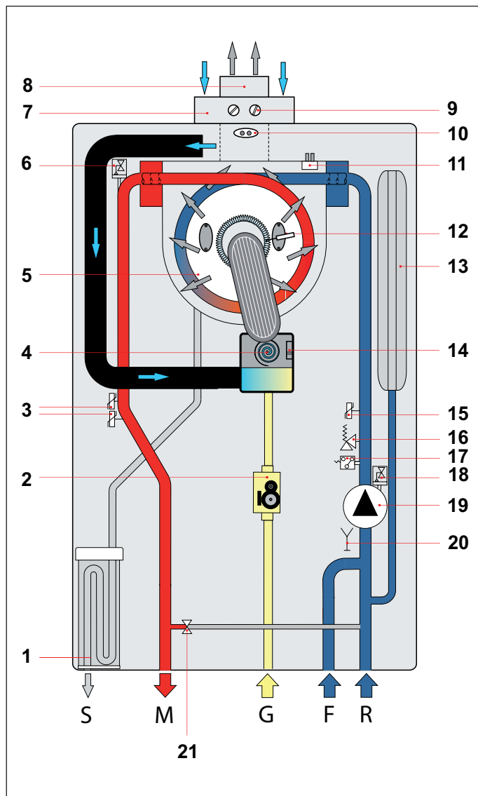
Εικ. 7 Υδραυλικό διάγραμμα μοντέλου KR
