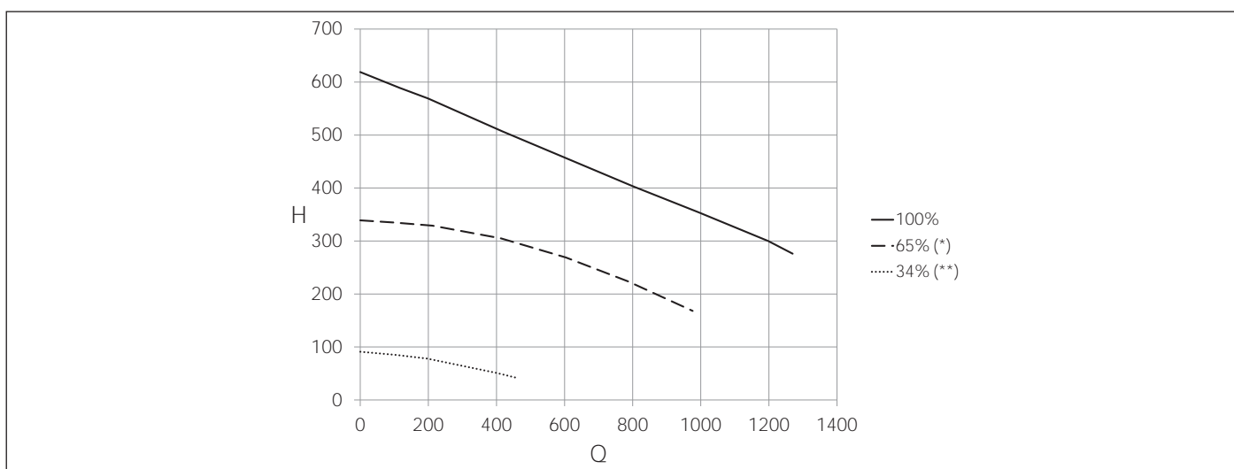
Εικ. 23 Διαθέσιμη αντίσταση KC-KR-KRB 32
